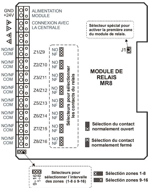
Figure 17. Configuration des bornes et des ponts de l'MR8.
